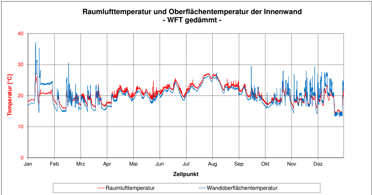
Abbildung 23 Vergleich Taupunkttemperatur der Raumluf / raumseitige Oberflächentemperatur – Wandflächentemperierung, gedämmt
