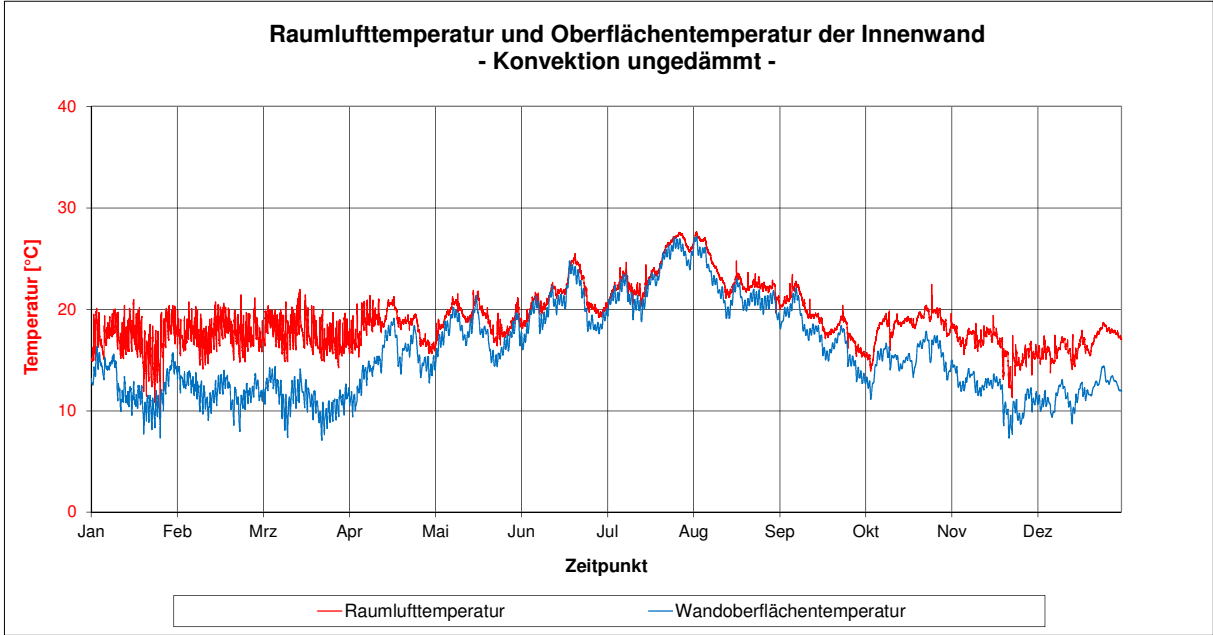
Abbildung 20 Vergleich Taupunkttemperatur der Raumluft / raumseitige Oberflächentemperatur – Konvektion, ungedämmt
