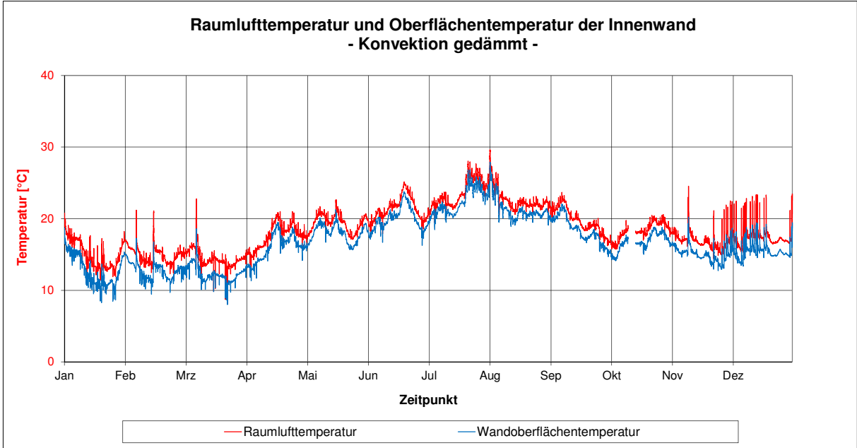
Abbildung 21 Vergleich Taupunkttemperatur der Raumluft / raumseitige Oberflächentemperatur – Konvektion, gedämmt
