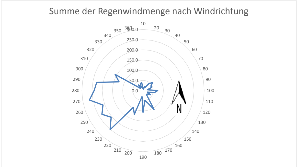
Abbildung 30 Produkt aus Regenmenge und Windgeschwindigkeit nach Himmelsrichtung am Standort Hamburg Fuhsbüttel (Berechnet auf Grundlage der Angaben des DWD)
