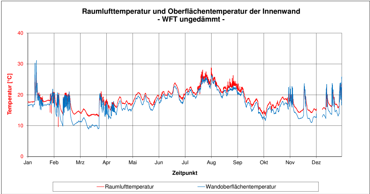
Abbildung 22 Vergleich Taupunkttemperatur der Raumluf / raumseitige Oberflächentemperatur – Wandflächentemperierung, ungedämmt
