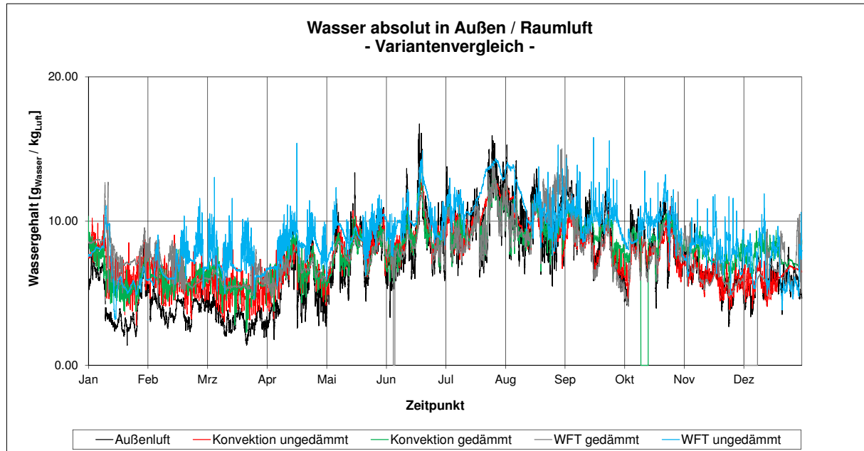
Abbildung 19 Vergleich der Wassermengen in der Außenluft und in der Raumluft
