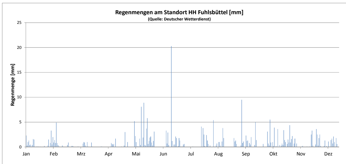
Abbildung 25 Niederschlagsmengen am Standort Hamburg Fuhlsbüttel (Quelle: DWD)
