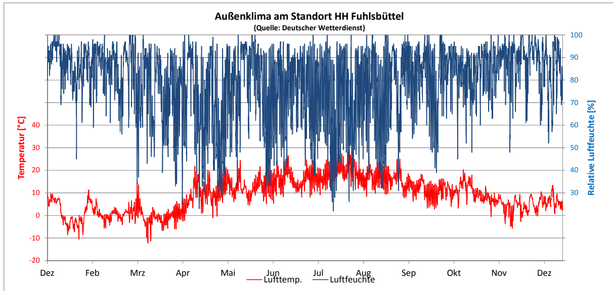
Abbildung 24 Außenklima am Standort Hamburg Fuhlsbüttel (Quelle: DWD)
