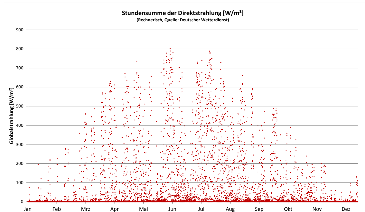
Abbildung 28 Stundensummen der Direktstrahlung am Standort Hamburg Fuhlsbüttel (Berechnet auf Grundlage der Angaben des DWD)
