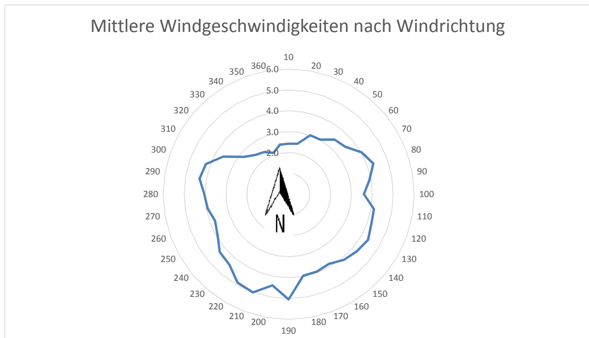
Abbildung 29 Mittlere Windgeschwindigkeiten [m/s] nach Himmelsrichtung am Standort Hamburg Fuhlsbüttel (Berechnet auf Grundlage der Angaben des DWD)
